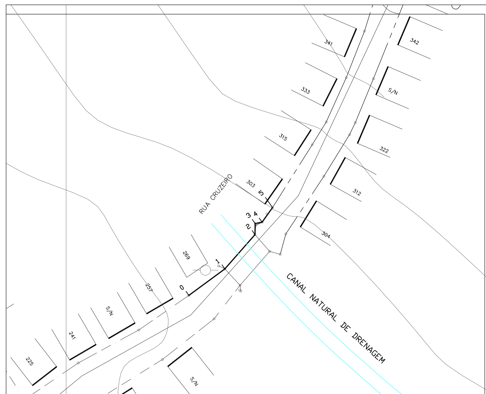
PLANTA ESC. 1:500
