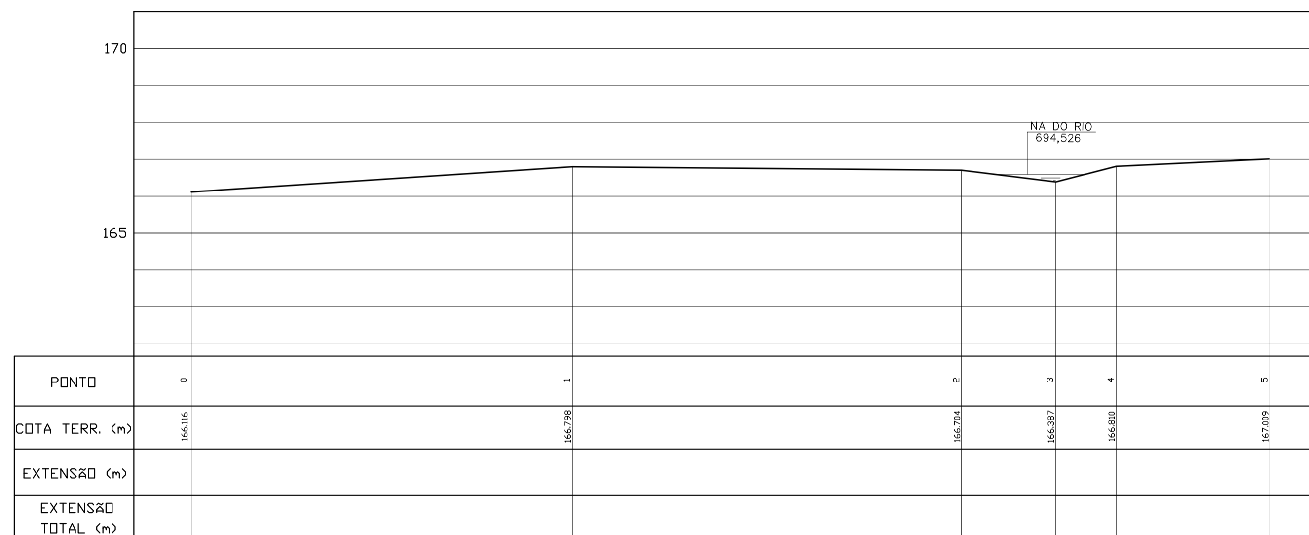
PERFIL ESC. 1:100
