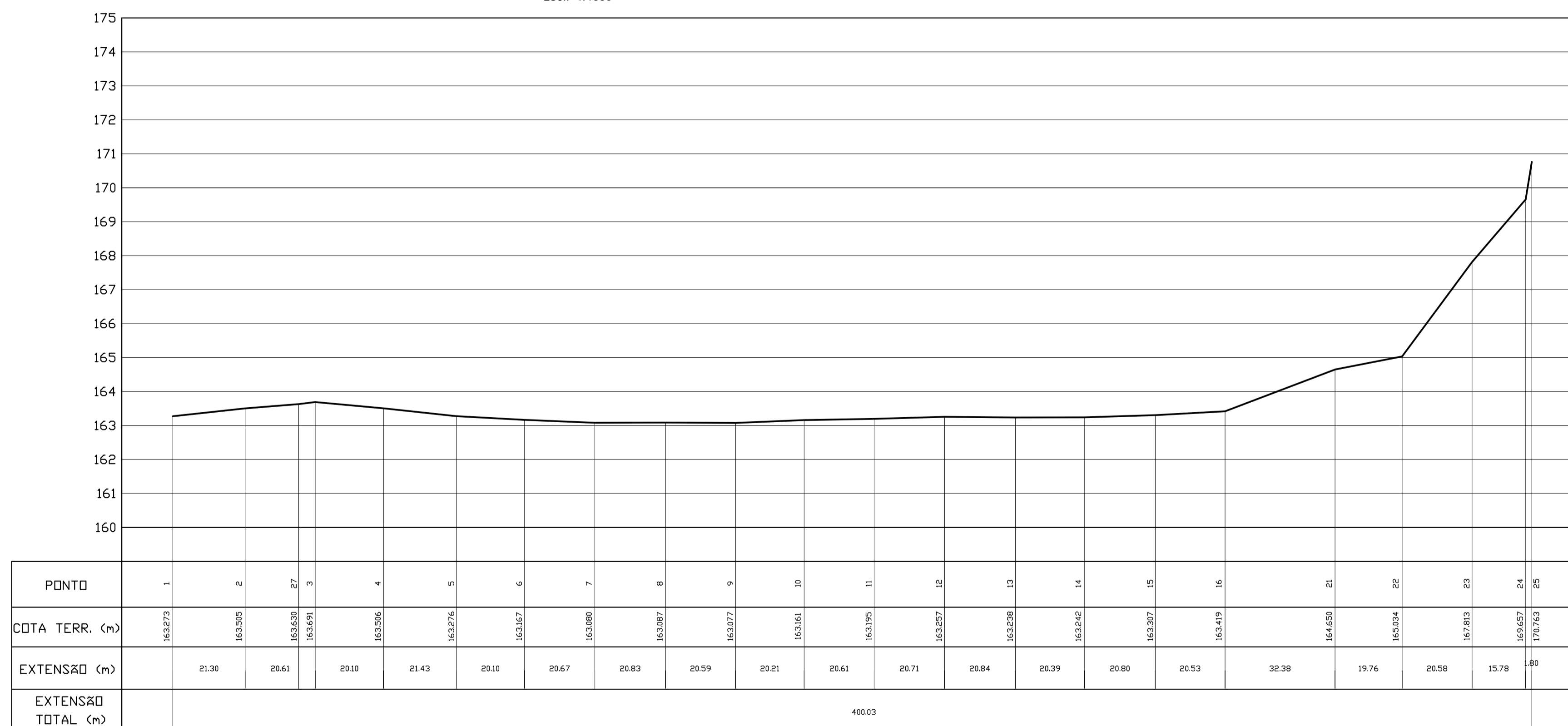
PERFIL-LONGITUDINAL ESC. HOR.: 1:1000 VER.: 1:100
