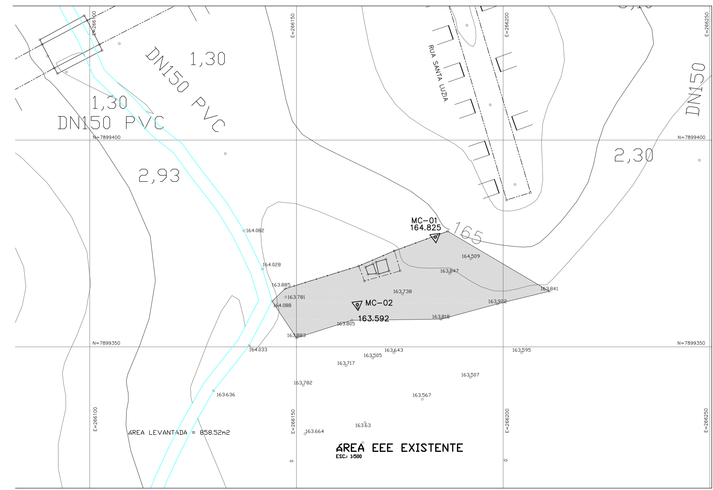
ÁREA EEE EXISTENTE ESC.: 1:500
