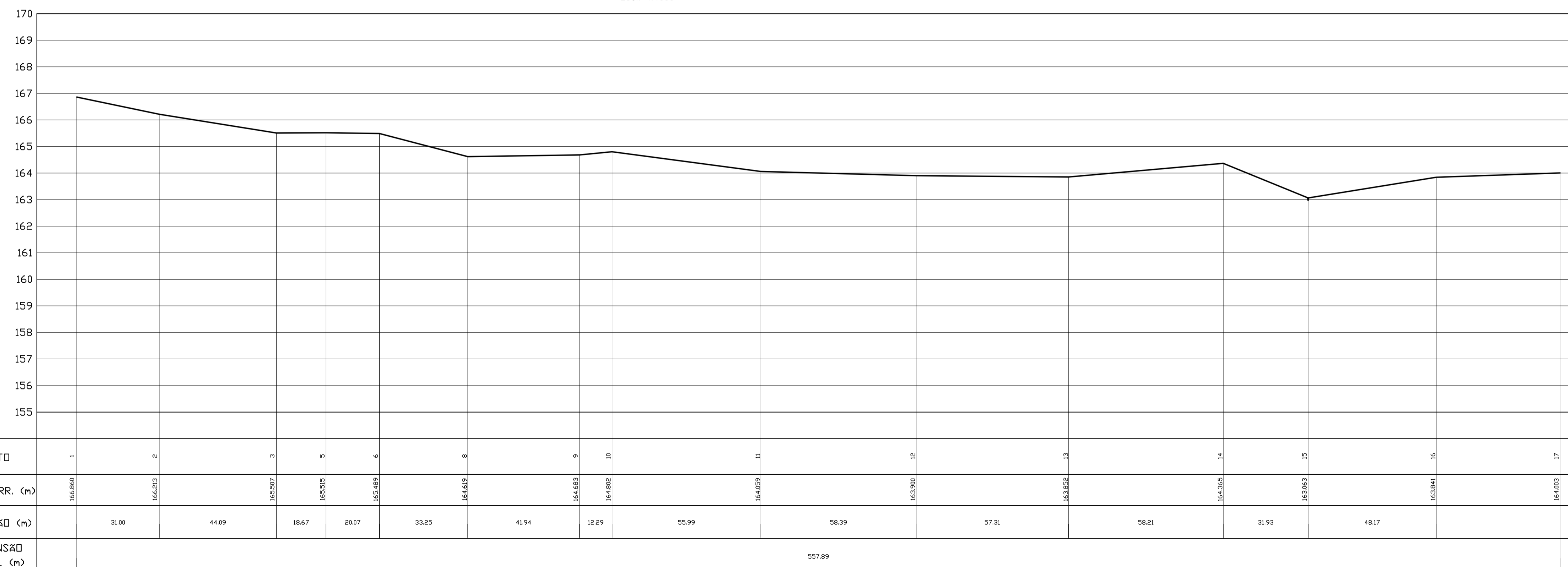
PERFIL—LONGITUDINAL ESC. HOR.: 1:1000 VER.: 1:100
