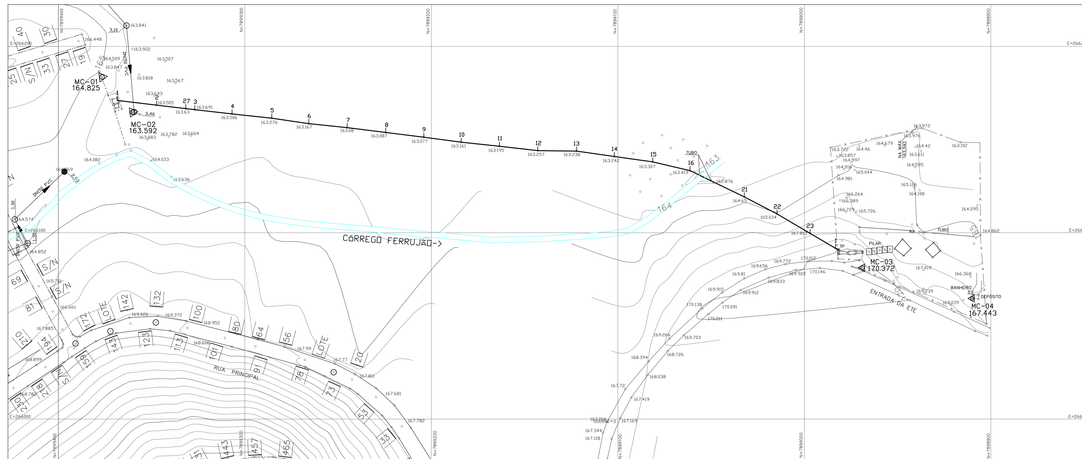
LINHA DE RECALQUE ESC.: 1:1000
