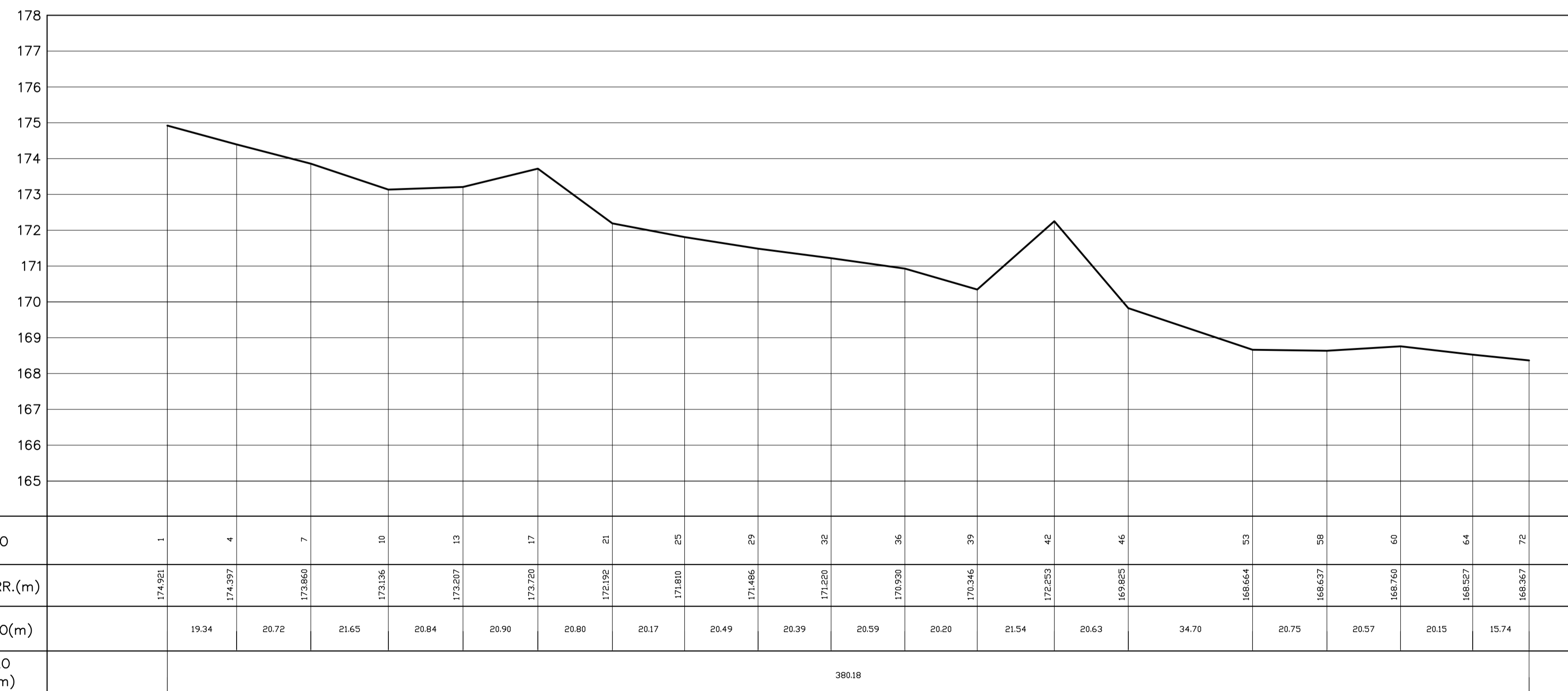
PERFIL-LONGITUDINAL ESC. HOR.: 1:1000 ESC. VER.: 1:100
