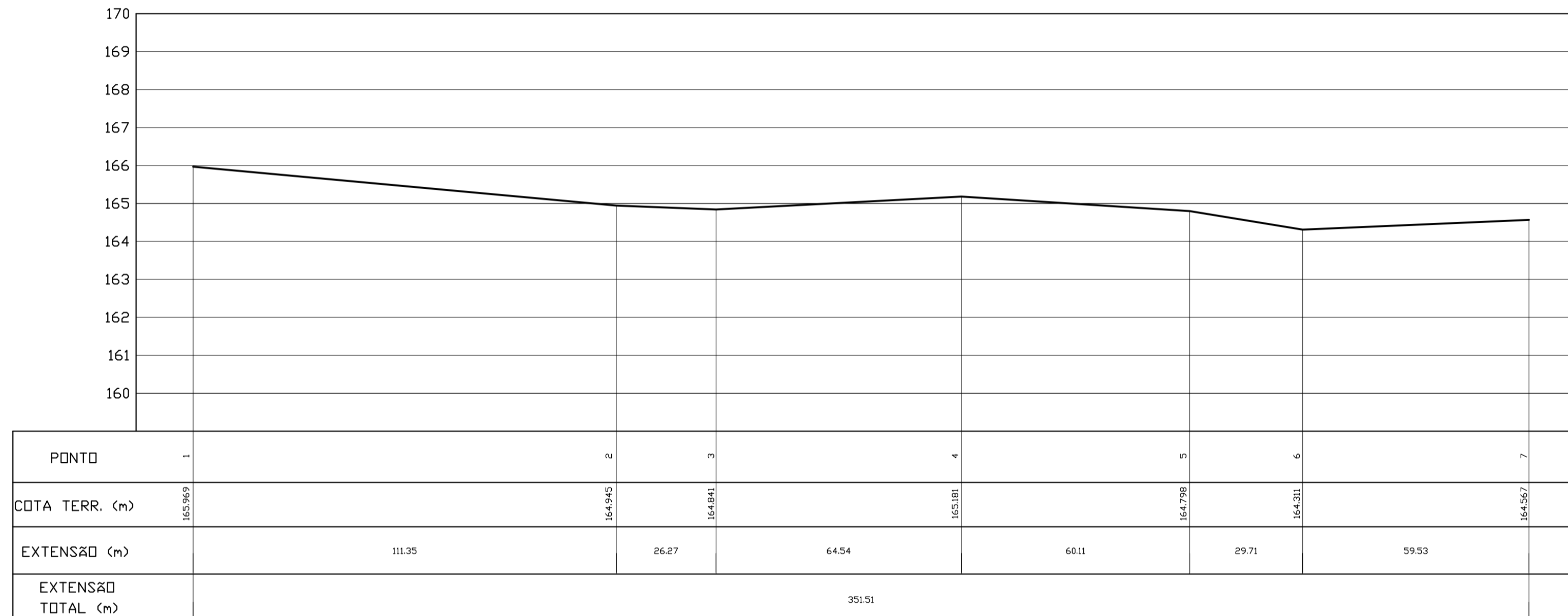
PERFIL—LONGITUDINAL ESC. HOR.: 1:1000 VER.: 1:100
