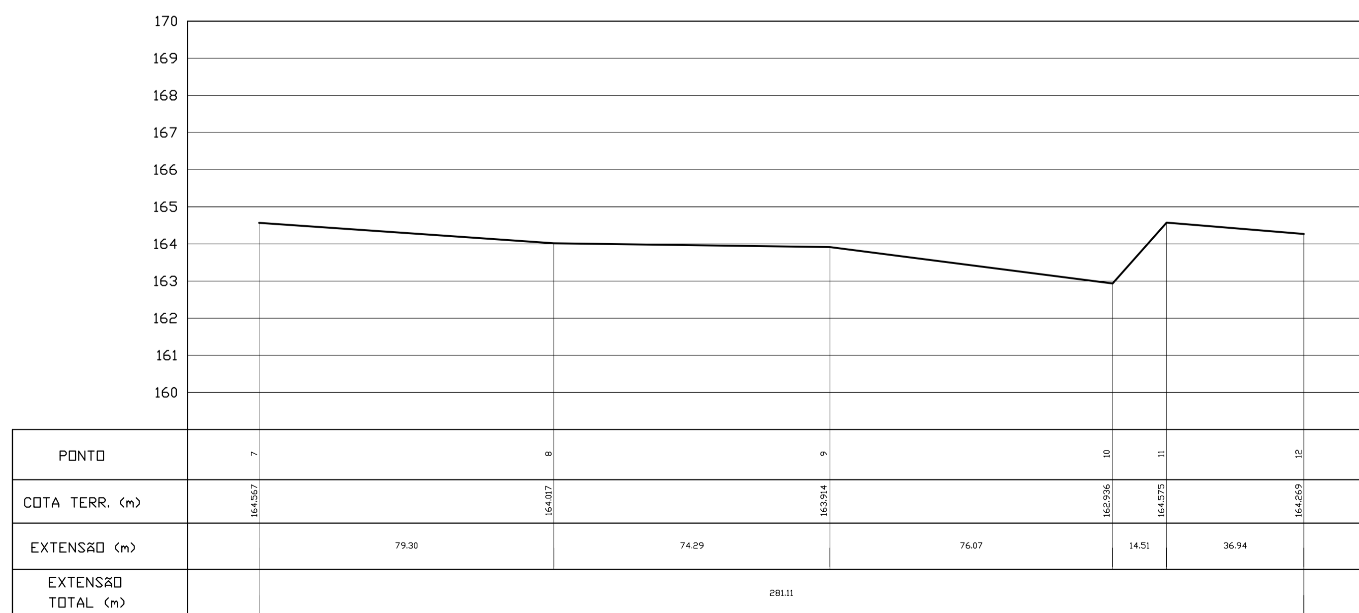
PERFIL—LONGITUDINAL ESC. HOR.: 1:1000 VER.: 1:100
